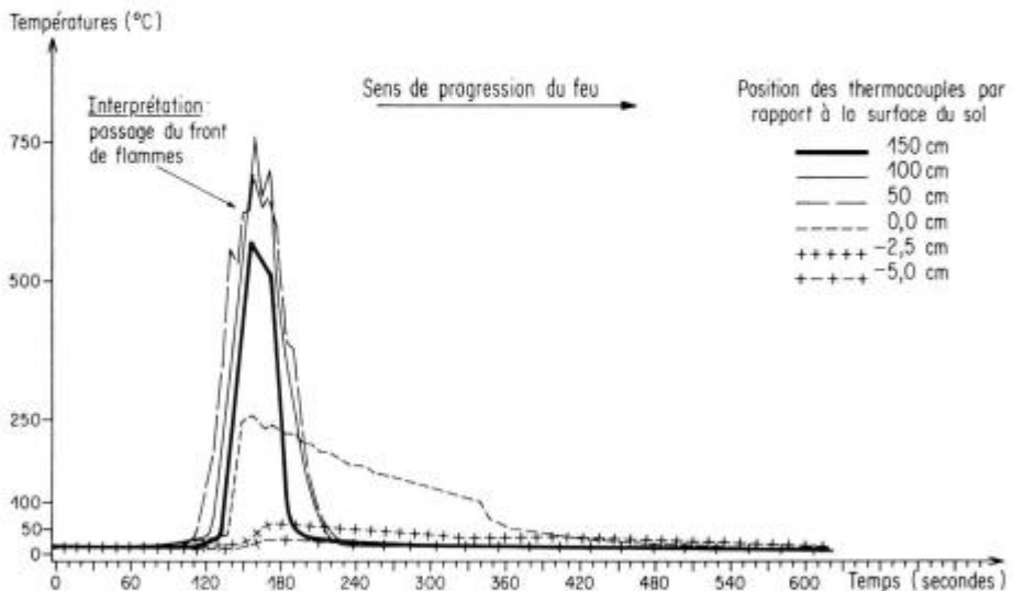
FIG. 3. — Courbes d'enregistrement des températures lors d'un feu d'« automne ». Végétation : 0,40 m de hauteur, 6 \text{ t} de MS. \text{ha}^{-1} ; vent : 2 \text{ m} \cdot \text{s}^{-1} ; hauteur du front de flammes : 0,70 m
